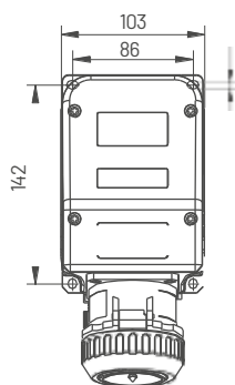
Tomada sobrepor
