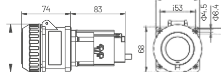
Tomada embutir
