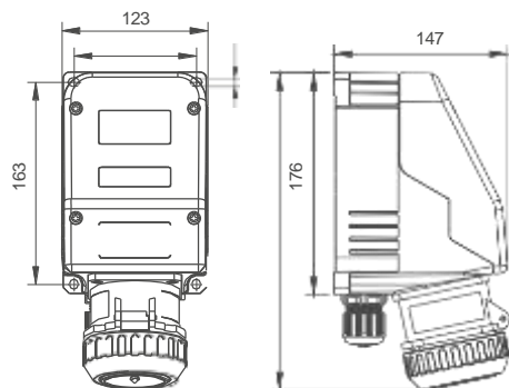
Tomada sobrepôr
