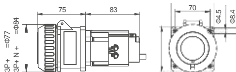
Tomada embutir
